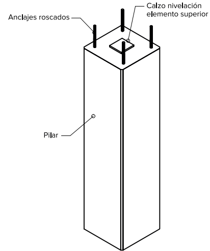
CABEZA PLANA CON ANCLAJES ROSCADOS (CABEZA STANDARD CONEXIÓN SUPERIOR)
