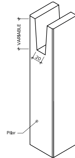
CABEZA PLANA CON HORQUILLA (APOYO STANDARD VIGAS PERALTADAS)
