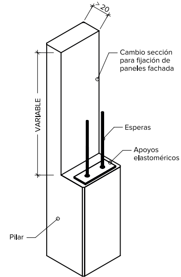
CABEZA CAMBIO SECCIÓN CON ESPERAS (APOYO STANDARD JACENAS FACHADA)
