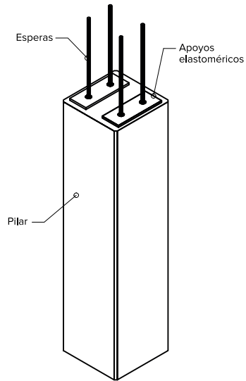
CABEZA PLANA CON ESPERAS (APOYO STANDARD JACENAS INTERMEDIAS)
