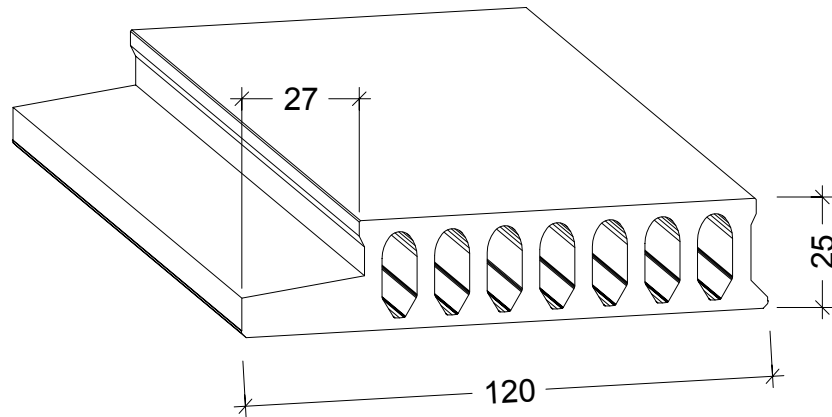
PLACA ALVEOLAR CORTAFUEGOS NPC-120/25
