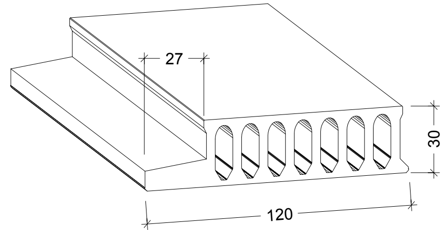
PLACA ALVEOLAR CORTAFUEGOS NPC-120/30
