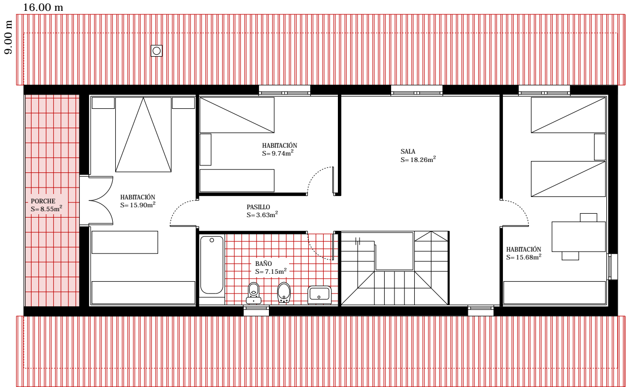
PLANTA PRIMERA VIVIENDA E: 1:100
