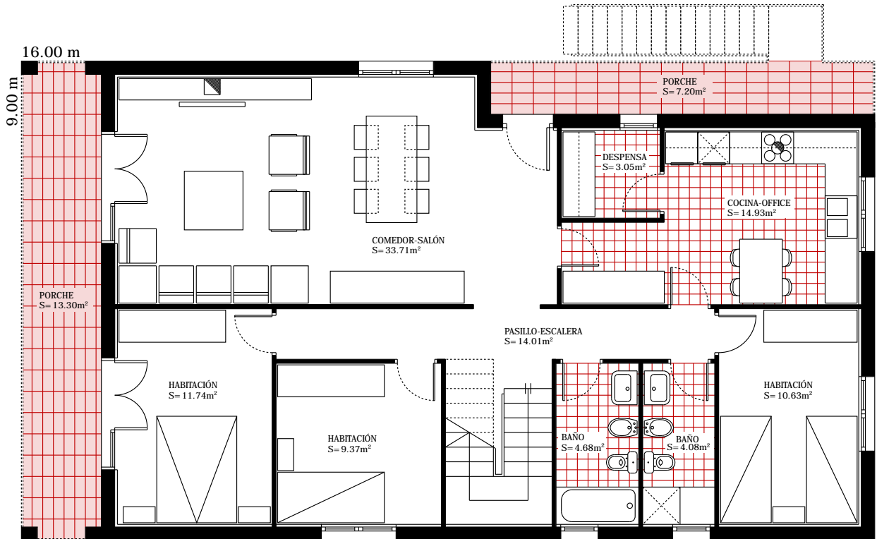
PLANTA BAJA VIVIENDA E: 1:100
